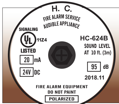
HC-624B 24 VDC
